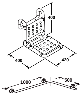
► Siège de douche J445801 A accrocher sur barre de maintien d'angle
